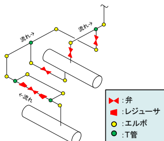
配管のアイソメ図
