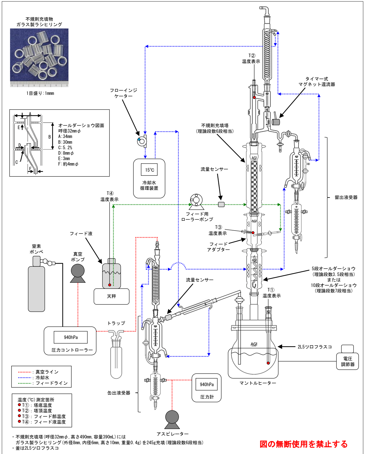
ガラス製蒸留装置イメージ図 (不規則充填塔+オーダーショーウ+フィードアダプターによる連続蒸留/大気圧系)
