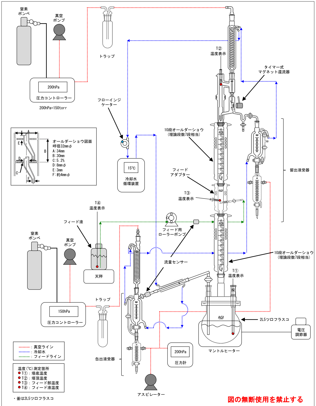
ガラス製蒸留装置イメージ図 (オールダーショウ×2本+フィードアダプターによる連続蒸留/減圧系)
